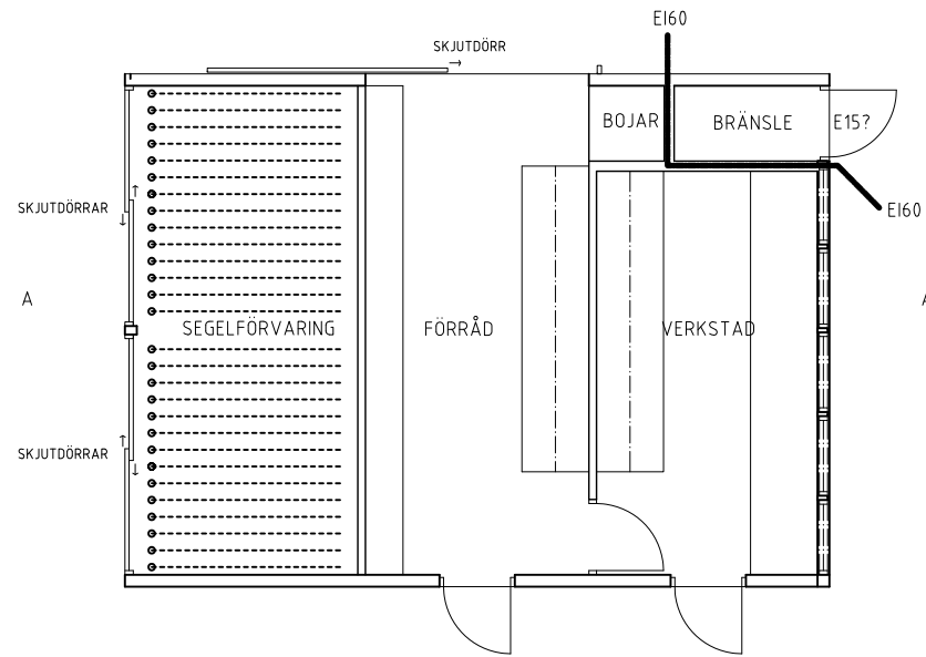
PLAN SKALA 1:100
